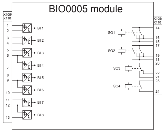
Figure 26. Optional BIO0005 module (slot X105)
