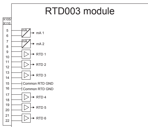
Figure 28. Optional RTD0003 module (slot X105)
