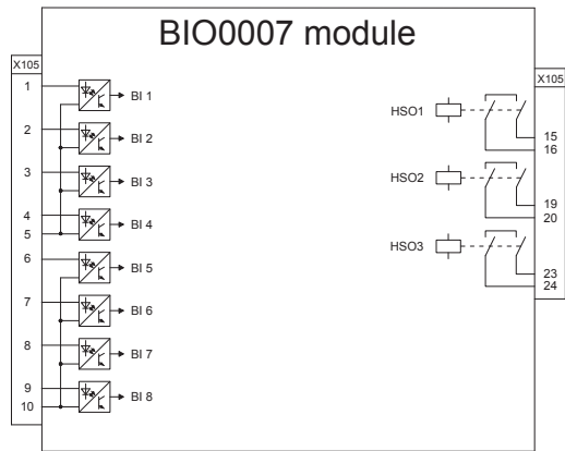
Figure 27. Optional BIO0007 module for fast outputs (slot X105)
