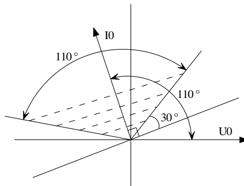
(图) 零序方向元件动作区域
