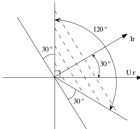
(图) 方向元件动作区域
