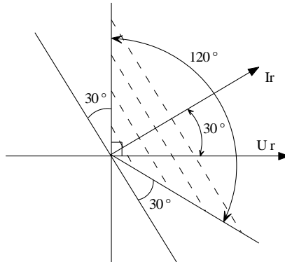
(图) 方向元件动作区域
