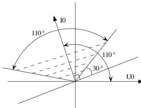
(图) 零序方向元件动作区域
